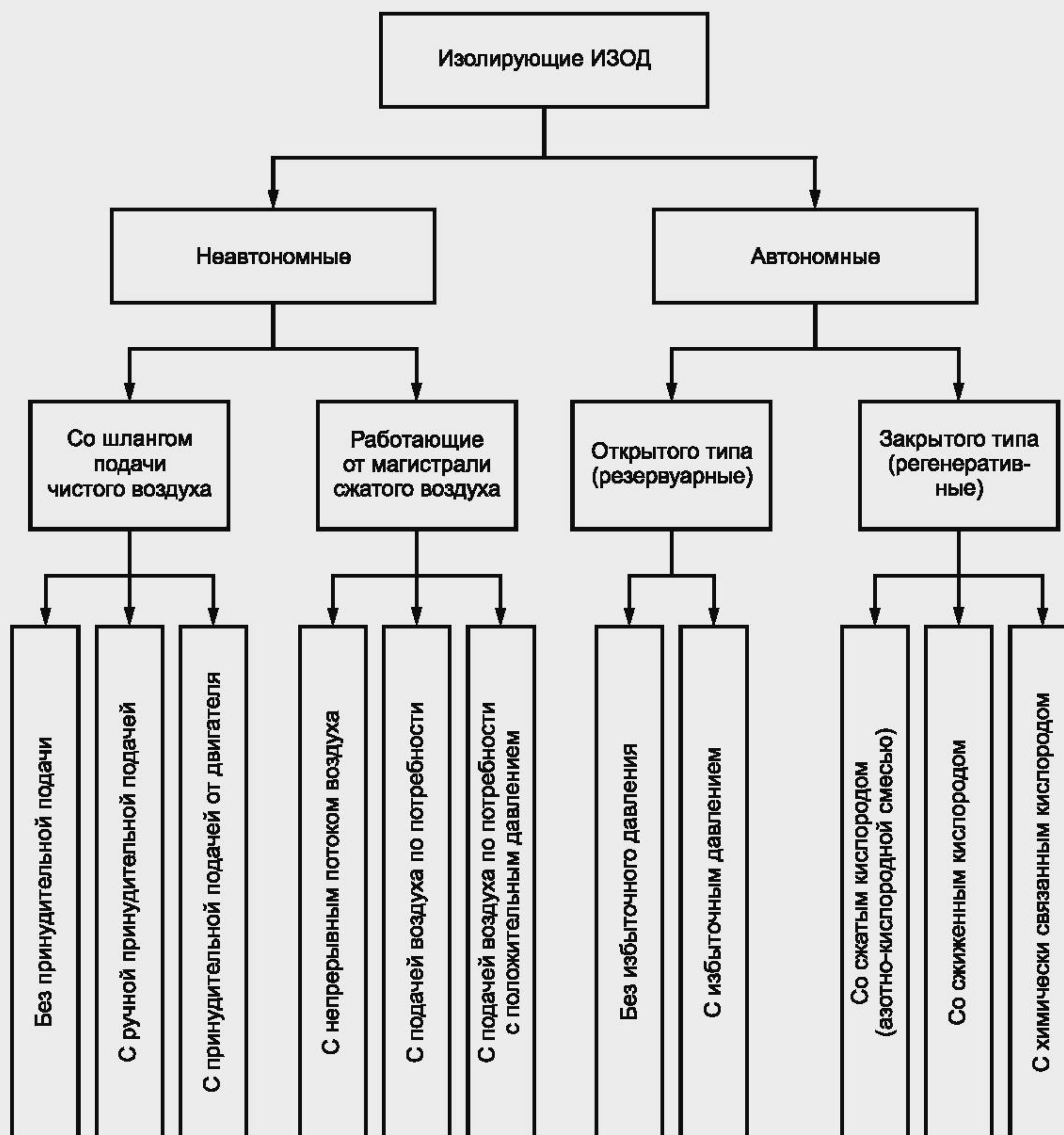
Рисунок 4 — Классификация изолирующих СИЗОД по конструкции и принципу действия
