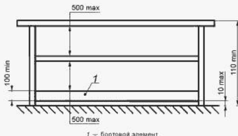
Рисунок 3 — Пример горизонтальных защитных ограждений
