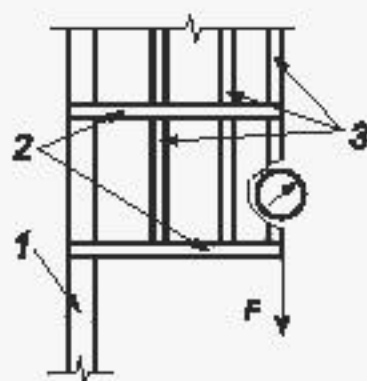
1 — тетива лестницы, 2 — дуга ограждения, 3 — продольная полоса ограждения
