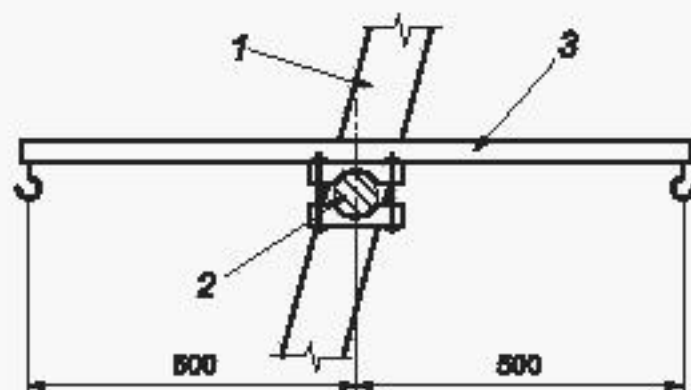
1 — тетива лестницы; 2 — ступень (перекладина) лестницы; 3 — двуплечий рычаг
