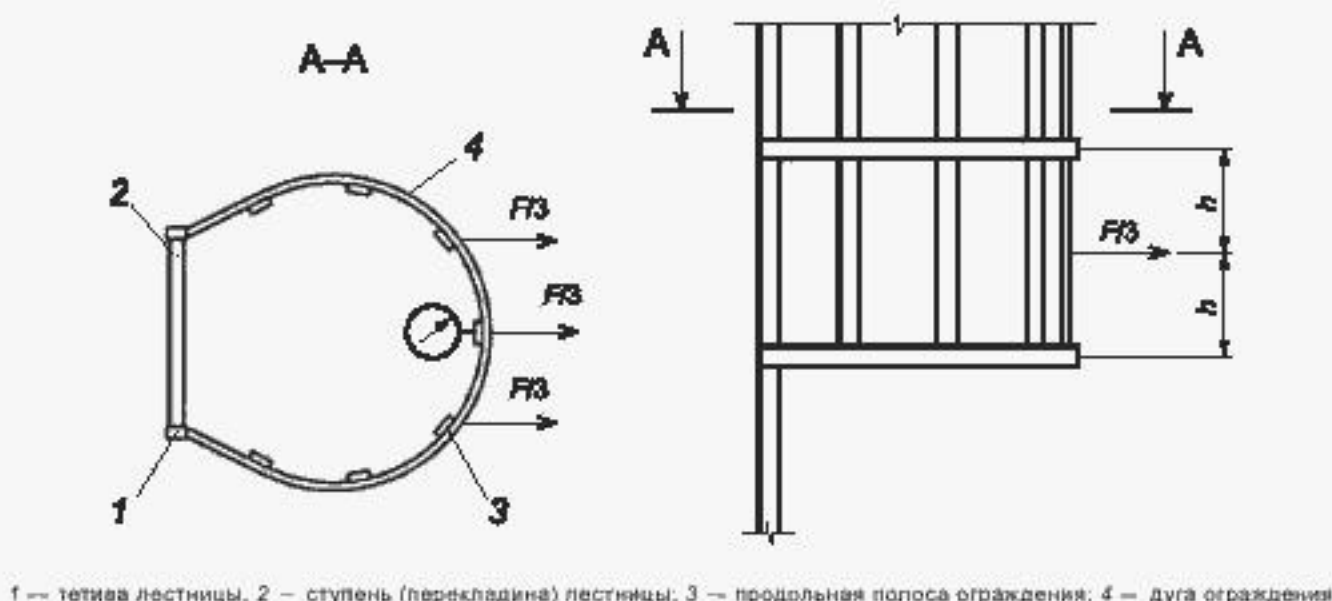
Рисунок 8 — Схема испытания ограждения навесной лестницы на прочность при воздействии горизонтальной статической нагрузки
