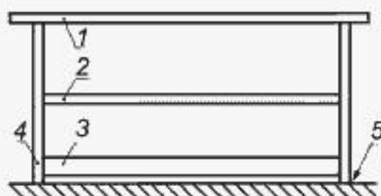
1 — поручень; 2 — ограждение для коленей; 3 — бортовой элемент; 4 — стойка; 5 — уровень настила пола
