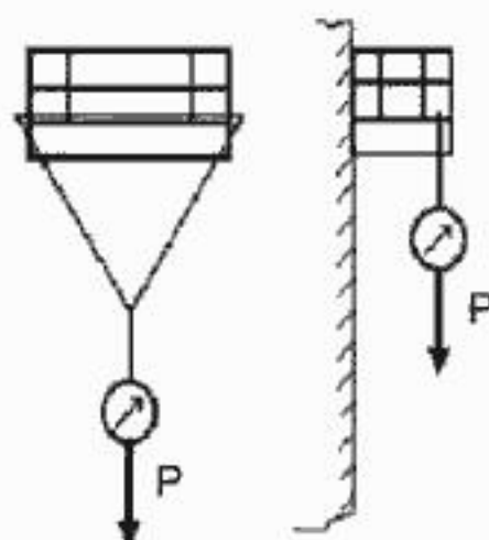
Рисунок Д.4 — Площадка
