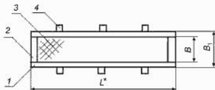
1 — балка; 2 — окантовочный элемент; 3 — настил; 4 — ребро
