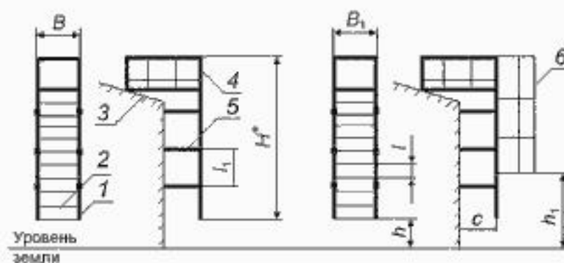
Рисунок Б.1 — Вертикальные лестницы
