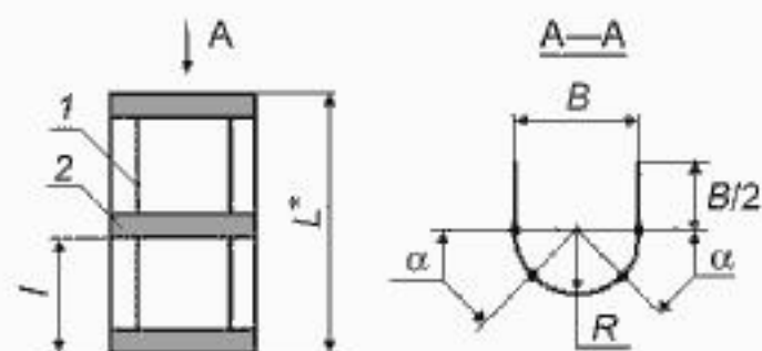
Рисунок Б.2 — Ограждения вертикальных лестниц
