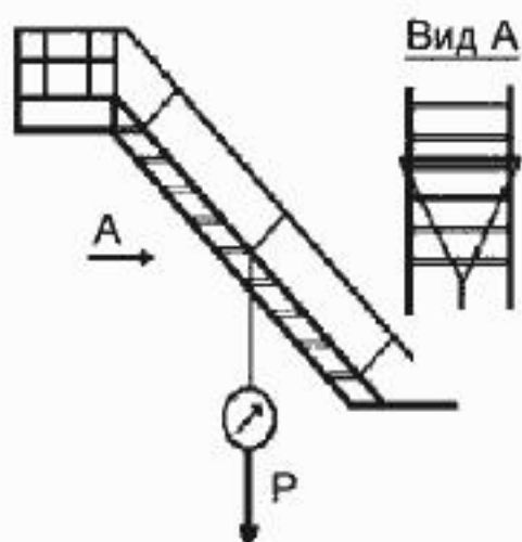
Рисунок Д.3 — Лестничный марш
