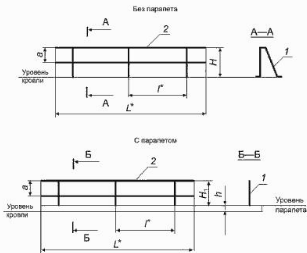
Рисунок Г.1 — Ограждения кровли
